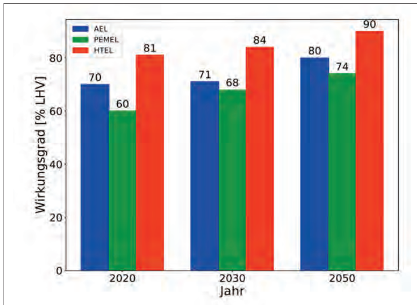
Abbildung 4.7: Prognostizierte Effizienzentwicklung der Elektrolysetechnologien [DLR- Wasserstoff als Fundament der Energiewende]
