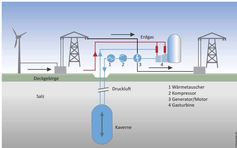
Abb. 3.3.1.3.1: Schema-Diabates-CAES-Kraftwerk | Abb: RENAC
