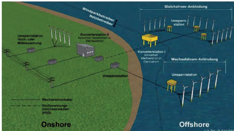
Abb. 3.1.6.2: Windenergie On- und Offshore und ihre Netzanbindung
