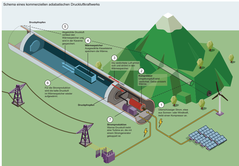
Abb. 3.3.1.3.2: Schema eines kommerziellen adiabatischen Druckluftkraftwerkes / Abb: Tages Anzeiger/ ALACAES
