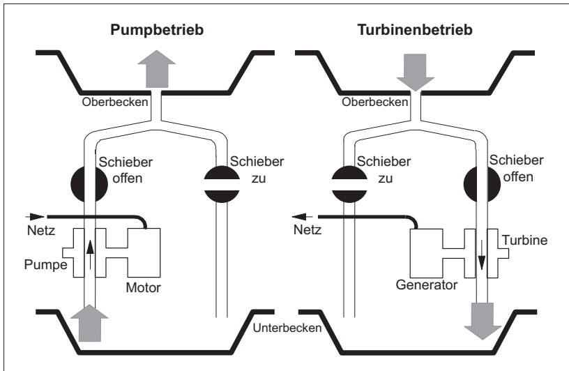
Abb. 3.3.1.1.1: Arbeitsweise eines Pumpspeicherwerkes | Quelle: Springer-Vieweg
