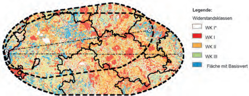
Abb. 5.5.3: Beispiel einer kombinierten Widerstandskarte im Maximalwertverfahren | Quelle: ILF
