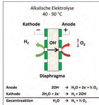
Abbildung 4.4: Alkalische Elektrolyse [DLR-Wasserstoff als Fundament der Energiewende]
