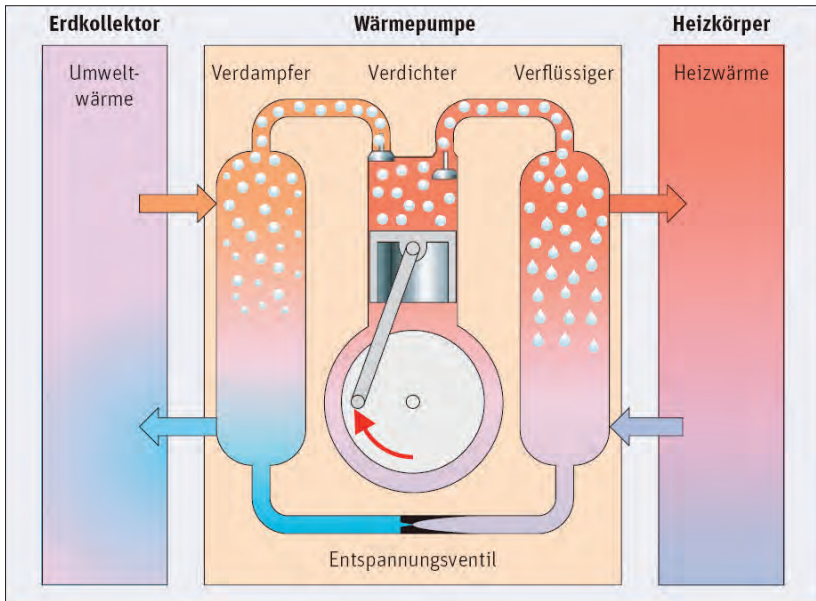
Abb. 3.1.7.1: Arbeitsprinzip einer Wärmepumpe | Quelle: Sunbeam-berlin.de
