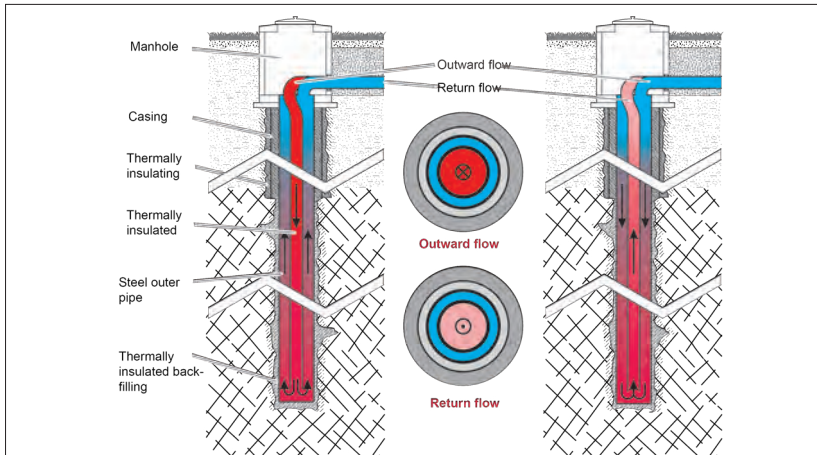
Abb. 3.1.7.3: Koaxiale Erdwärmesonde für den Einsatz in mitteltiefen Erdwärmesondenspeichern (links: Beladungsphase, rechts: Entladungsphase) | Quelle: Bär et al. 2015
