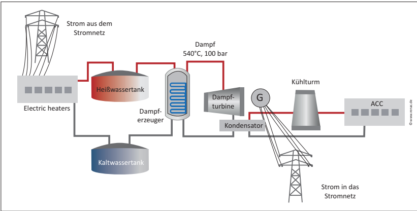
Abb. 3.3.2.4: Elektrisches Wärmespeichersystem mit Rückverstromung | Quelle: TSK Flagsol Engineering GmbH | Abb: RENAC
