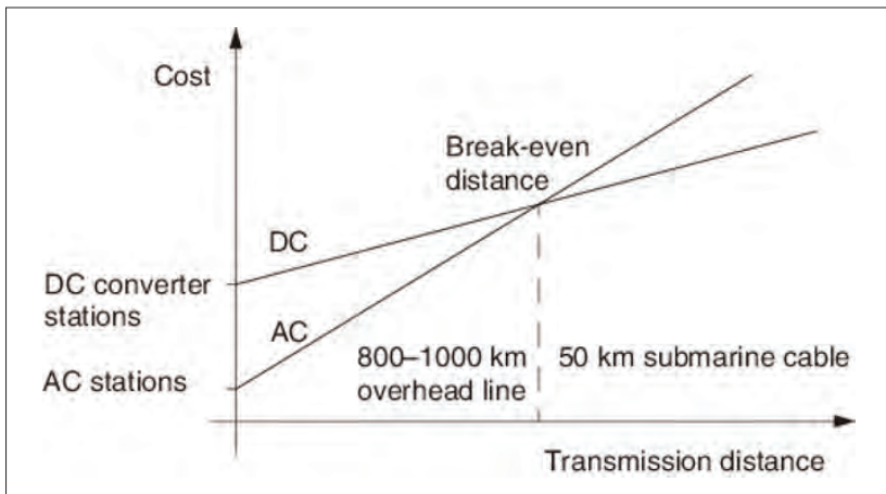
Figure 3.2.1.5.1: Breakeven-Distanz für HGÜ | Source: P. Schavemaker & L. van der Sluis 2008).
