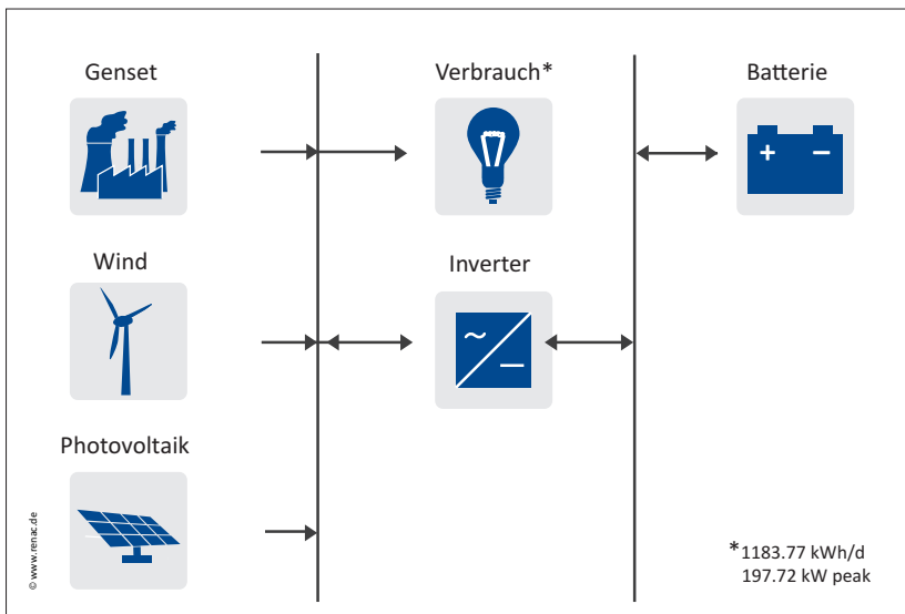
Abb. 3.1.9.2.2: Beispiel für die schematische Modellierung von Hybridsystem | Quelle: Homer Energy| Abb.: RENAC
