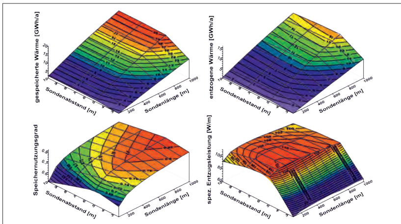
Abb. 3.1.7.6: Einfluss von Sondenlänge und Sondenabstand auf verschiedene Speicherleistungsindikatoren, dargestellt für einen exemplarischen Speicher aus 37 Erdwärmesonden im 30. Betriebsjahr | Quelle: Welsch et al. 2015
