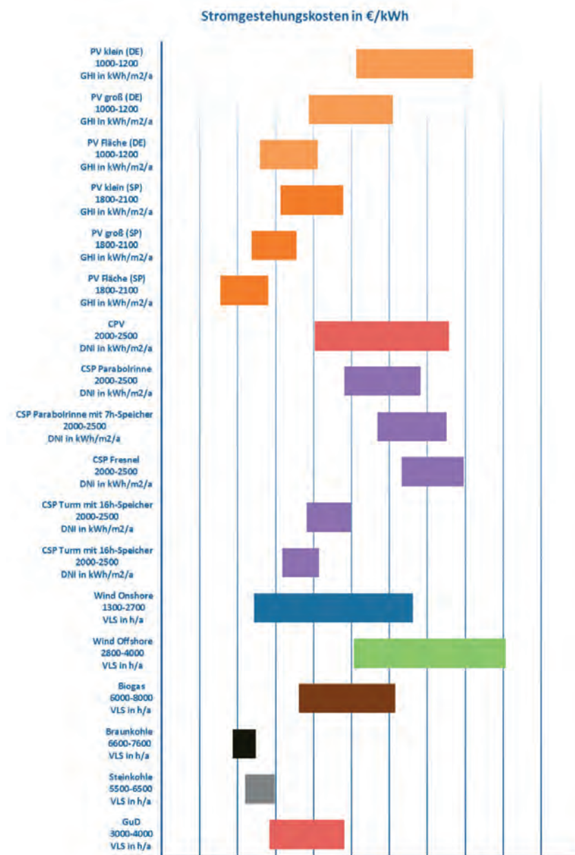
Abb. 6.1.2: Die Zahlen unter der jeweiligen Technologie geben die jährlich geleisteten Volllaststunden an – bei Solaranlagen ist es die Stromausbeute pro Quadratmeter / Quelle: Fraunhofer ISE
