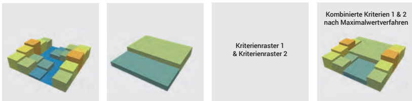
Abb. 5.5.2: Maximalwertverfahren von Widerstandswerten | Quelle: ILF
