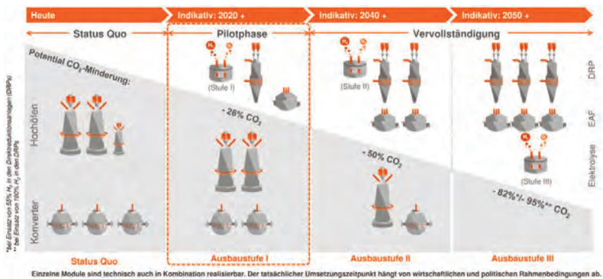
Abbildung 4.12: Stufenweise Umstellung auf eine H 2 -basierte Stahlerzeugung (Projekt SALCOS) 23
