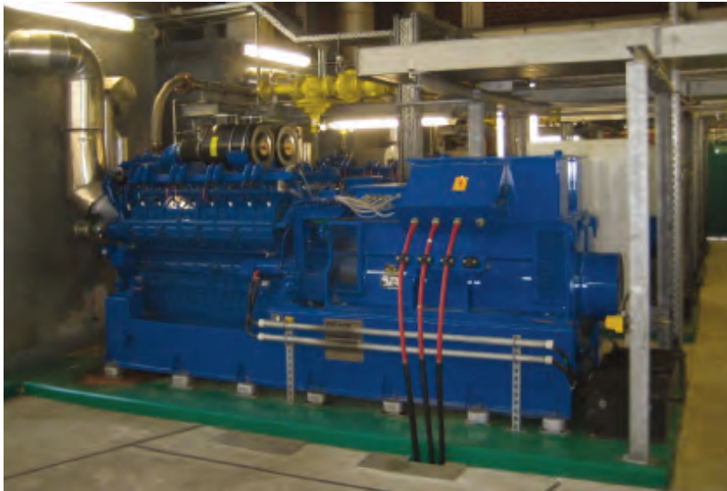
Abb. 3.2.4.4.1: Moderne Gas-KWK-Anlage Quelle: Dr. Born – Dr. Ermel GmbH
