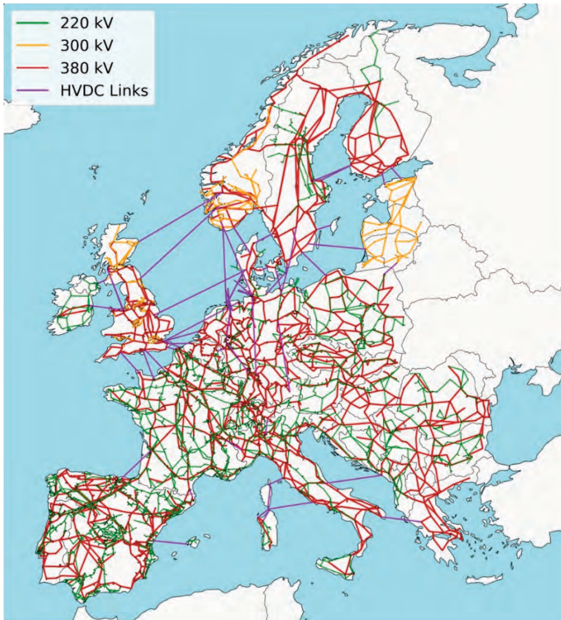
Figure 3.2.1.5.2: Elektrische Stromnetze in Europa.
