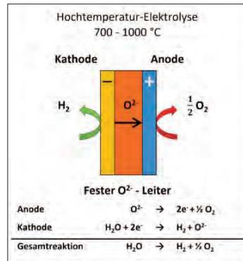
Abbildung 4.6: Hochtemperatur-Elektrolyse [DLR- Wasserstoff als Fundament der Energiewende]
