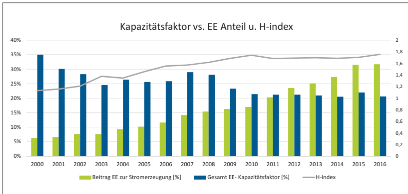
Abb. 3.1.1: Zeitliche Entwicklung des erneuerbaren Energienanteils an der Stromerzeugung, des Kapazitätsfaktors und des H-Index für Deutschland | Quelle: [2]
