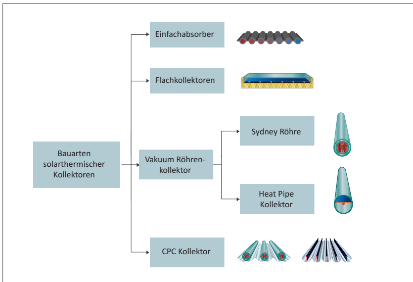
Abb. 3.1.1.1 Kollektorbauarten | Quelle: Fa. SOLID, Graz, Österreich
