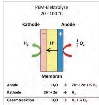
Abbildung 4.5: PEM-Elektrolyse [DLR-Wasserstoff als Fundament der Energiewende]
