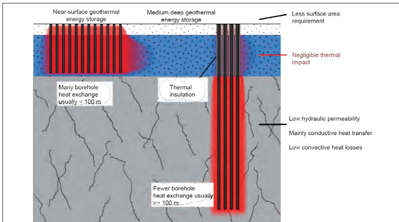
Abb. 3.1.7.4: Schematischer Vergleich des thermischen Einflusses auf Grundwasserleiter oberflächennaher und mitteltiefer Erdwärmesondenspeicher | Quelle: Welsch et al. 2015
