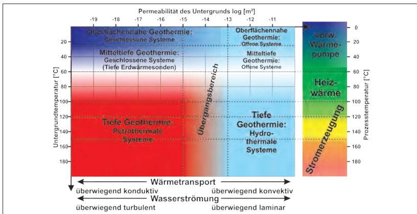
Abb. 3.1.7.2: Definitionsmöglichkeiten für geothermische Nutzsysteeme in Abhängigkeit von der Lagerstätten-Permeabilität und der Erschließungsteufe | Quelle: Sass 2012
