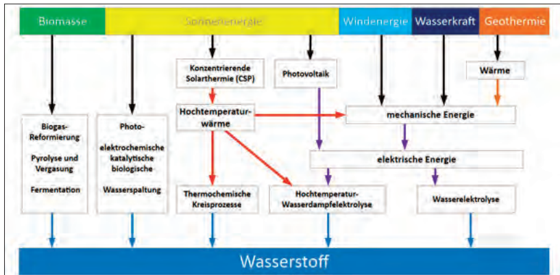
Abbildung 4.3: Pfade der Wasserstoffproduktion aus erneuerbaren Energien [DLR-Wasserstoff als Fundament der Energiewende]
