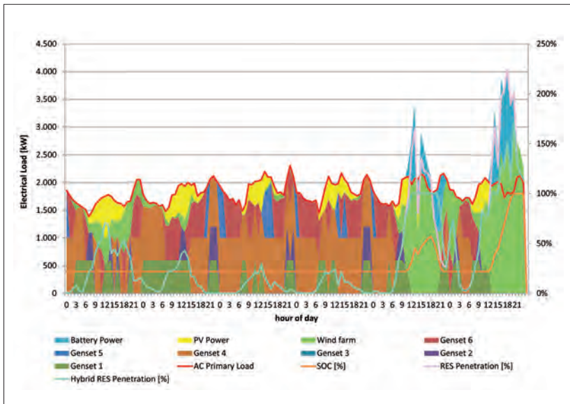
Abb. 3.1.9.2.1: Beispiel für stündliche Simulationsergebnisse eines Hybridsystems aus Windkraftanlagen, PV, Batterien und Diesellaggregaten | Quelle: Lahmeyer
