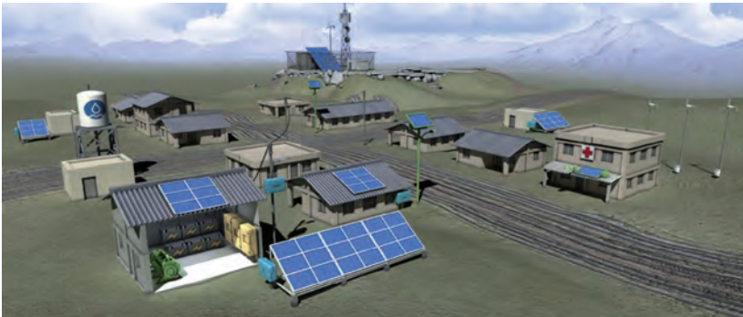
Abb. 3.2.1.3.1: Beispiel einer Minigrid-Anlage mit dezentraler PV-Stromerzeugung, Windkraftanlagen, Batterien, einem Dieselgenerator und einem kleinen Verteilungsnetz. Zusätzlich ist hier ein großer Wasserspeicher zu sehen. Die Pumpe für den Wasserspeicher dient als Beispiel für eine zeitlich verlagerbare Last, die Teil eines integrierten Steuersystems sein kann, das auch das Nachfragemanagement (Demand-Side-Management) umfasst. | Quelle: http://www.ennera.com/en/detail-solution/minigrids
