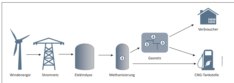
Abb. 3.2.2.1: Speicherung und Verteilung von erneuerbaren Energien | Quelle: RENAC
