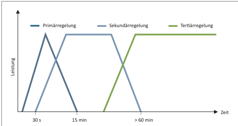
Abb. 3.3.3.2.4: Aufbau der drei Regeneurmermärkte – Im Primärregelungsmarkt müssen Anbieterinnerhalb von 30 s positive oder negative Regelleistung zur Verfügung stellen und maximal 15 min erbringen. | Quelle: Younicos | Abb. RENAC
